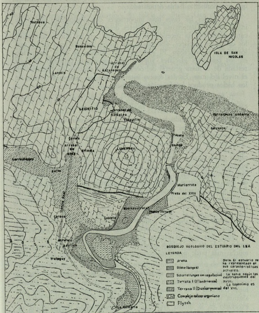
Figura 1.—Bosquejo geológico de la ría del Lea. La desembocadura, como debía de encontrarse a principios del XVIII.
